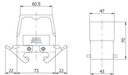
29175 29175S UZATMA GÖVDE-3 (M.Contalı) Hood (W.Locker&Seal)
