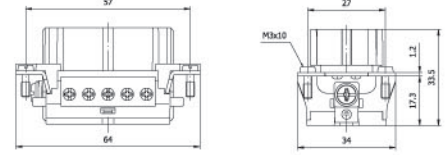
29174 UZATMA GÖVDE-3 Hood
