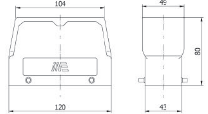
29179 29179S UZATMA GÖVDE-3 (M.Contalı) Hood (W.Locker&Seal)
