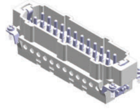
29025 FİŞ ÇEKİRDEK (1-24) Male Insert (1-24)
