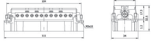
29178 UZATMA GÖVDE-3 Hood
