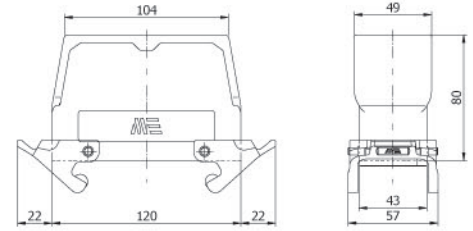
29179 29179S UZATMA GÖVDE-3 (M.Contalı) Hood (W.Locker&Seal)
