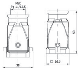
UZATMA FİŞ GÖVDE Hood For Male Insert
