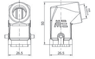
EĞİK FİŞ Hood With Male Insert (Angled)
