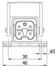
EĞİK FİŞ GÖVDE Hood For Male Insert (Angled)
