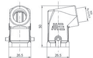
EĞİK FİŞ GÖVDE Hood For Male Insert (Angled)
