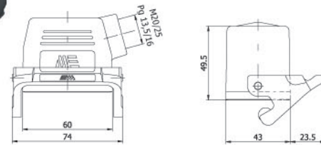
29132 UZATMA GÖVDE-2 (Yandan Girişli - M. Contalı) Hood (Side Entry-W.Locker & Seal)
